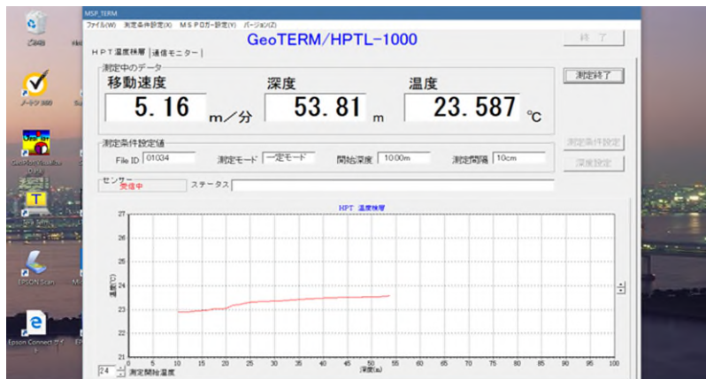
高分解能温度検層時における測定画面例
