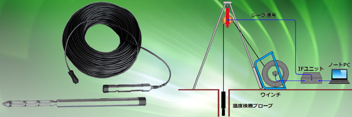
GeoHPT-1000 高分解能水温計
