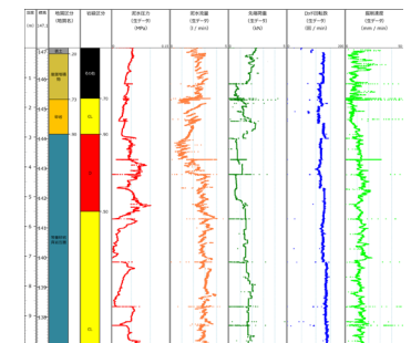
掘削時の物理値を示したグラフ
