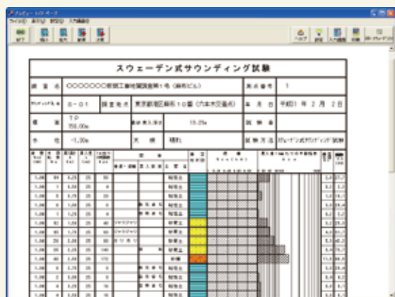
▲ スウェーデン式サウンディング試験柱状図
