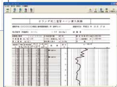
▼ オランダ式二重管コーン貫入試験
