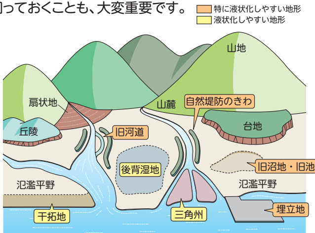
液状化しやすい地形
