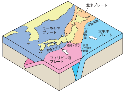
日本列島周辺のプレート
