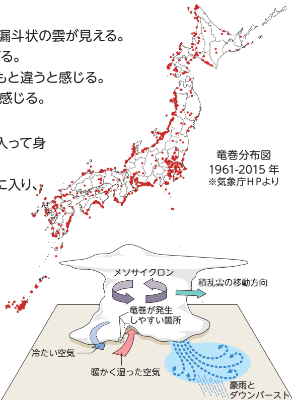
スーパーセルの模式図
