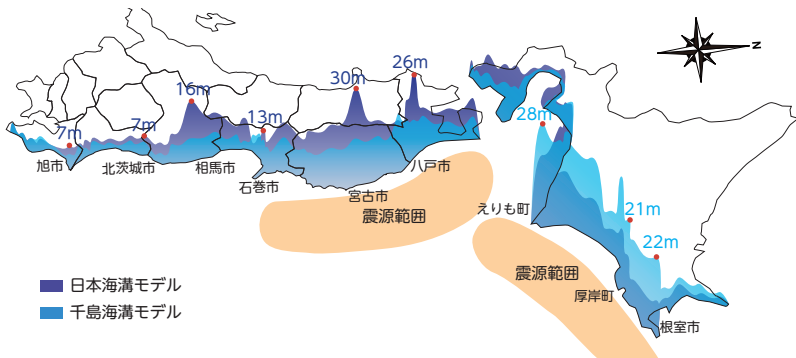
想定される沿岸での津波の高さ
