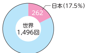
マグニチュード 6.0 以上の地震回数 (2010年～2019年)
