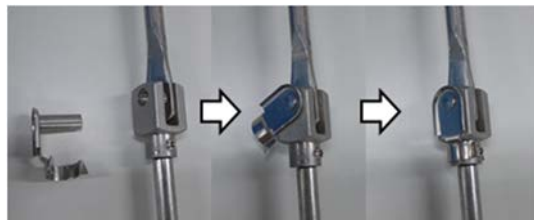
ピン差し込み → レバーロック
