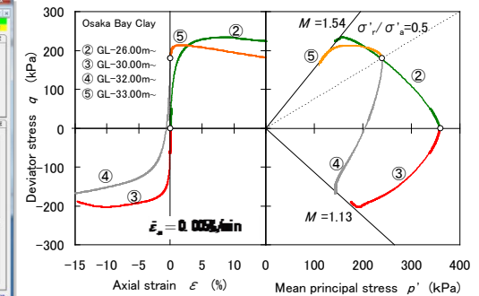
結果例 (等方・異方圧密 圧縮・伸張試験)
