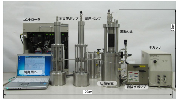
試験装置の全景
