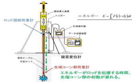
iPDCの測定装置の概要
