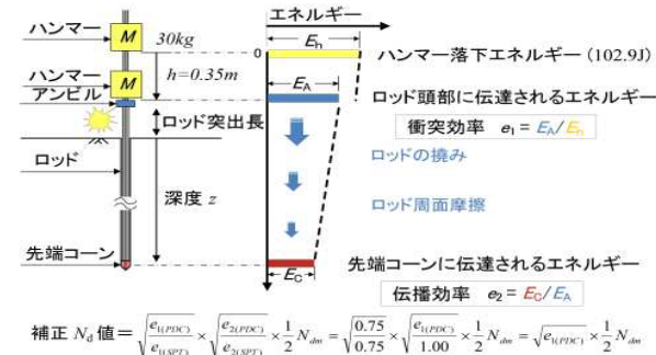
iPDC計測原理
